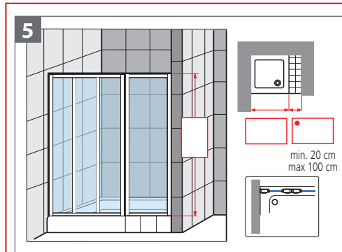
Fissaggio in linea / In-line fixing
