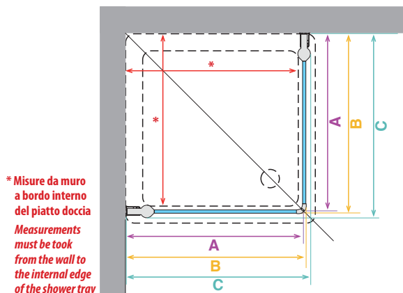
ref. 2 Giada 2G Cabina doccia angolare a 2 battenti Corner entry enclosure, 2 hinged doors
