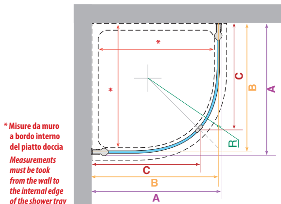
ref. 1 Giada R Cabina doccia angolare a 2 battenti Quadrant shower enclosure, 2 hinged doors
