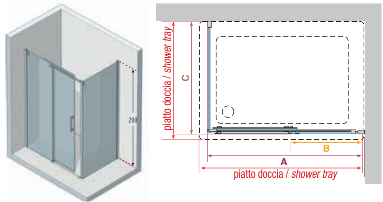
ref. 4 Diamanti 2P+F - Porta doccia a 2 ante, 1 scorrevole + 1 fissa con parete fissa laterale / 2 section door, 1 sliding + 1 fixed con parete fissa laterale
