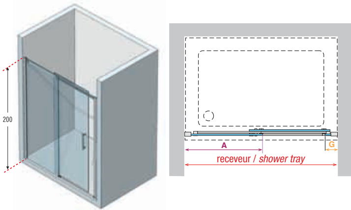
ref. 3 Diamanti 2P - Porte à 2 panneaux dont 1 coulissant en niche / 2 section door, 1 sliding + 1 fixed for recess
