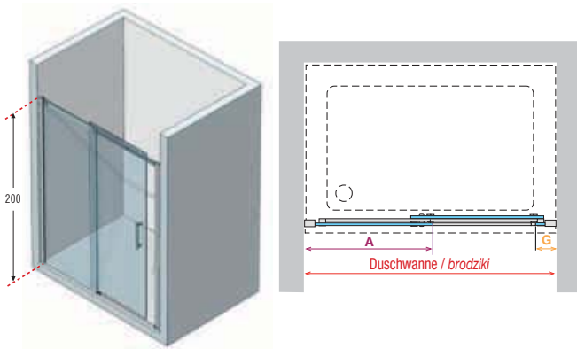
ref. 3 Diamanti 2P - Schiebetür (mit Festteil) Drzwi przesuwne ze ścianką stałą
