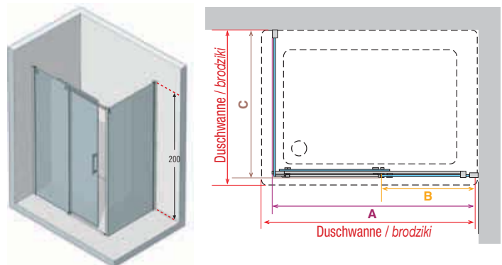
ref. 4 Diamanti 2P+F - Schiebetür (mit Festteil) und Seitenwand Drzwi przesuwne ze ścianką stałą + ścianka boczna F
