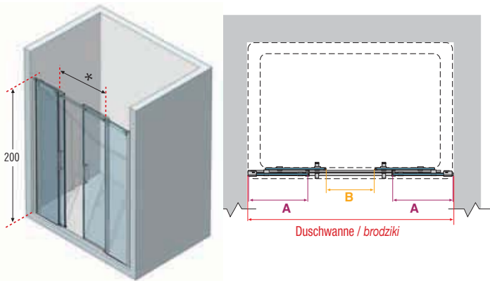
ref. 5 Diamanti 2A - Doppelte Schiebetür mit 2 Festteilen für Nischen- einbau / Podwójne drzwi przesuwne z 2 ściankami stałymi we wnęce
