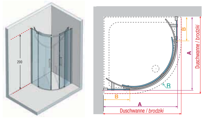
ref. 2 Diamanti R - Runddusche Kabina półokrągła
